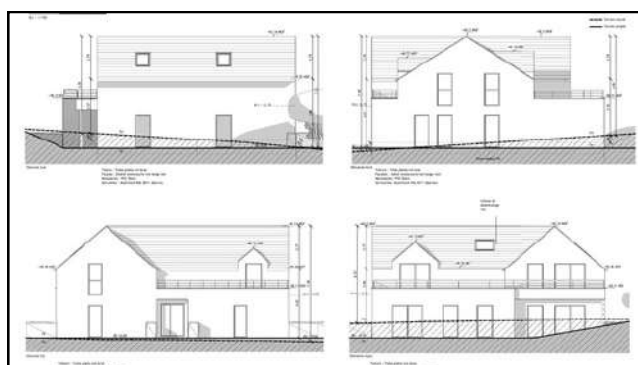
Pièce graphique du permis de construire
